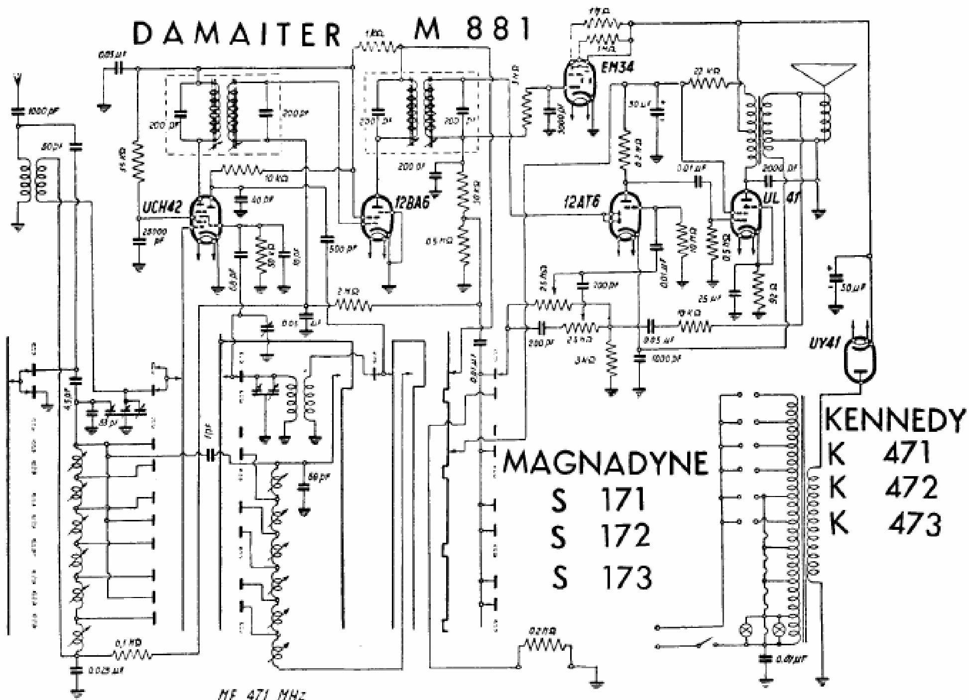
MAGNADYNE RADIO - Modd. S 171, S 172 e S 173, modd. Kennedy K 471, K 472 e K 473 e mod. Damaiter M 881. Gamma onde medie e sei bande allargate a onde corte (49, 41, 31, 25, 19 e 16 m.). Media frequenza 471 kc/s. Controllo di volume con compensazione dei toni bassi, a reazione inversa.
